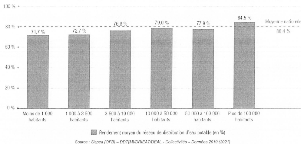
Graphique n° 1 : le rendement moyen des réseaux selon la taille des services (données 2019)
